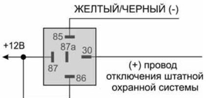
Подключение к (+) проводу снятия штатной сигнализации с охраны с использованием дополнительного реле
