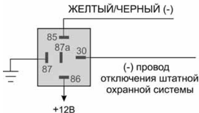
Подключение к (-) проводу снятия штатной сигнализации с охраны с использованием дополнительного реле
